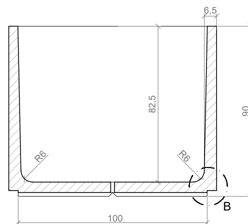
SECCION A-A' / SECTION A-A'
