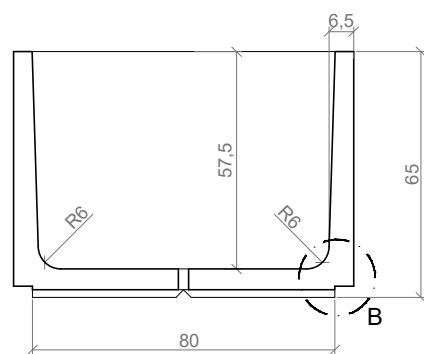
SECCION A-A' / SECTION A-A'
