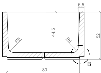
SECCION A-A' / SECTION A-A'
